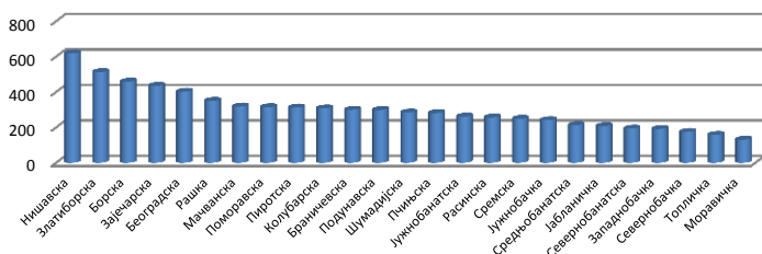
Специфична потрошња воде у насељима (л/ст/дан)
